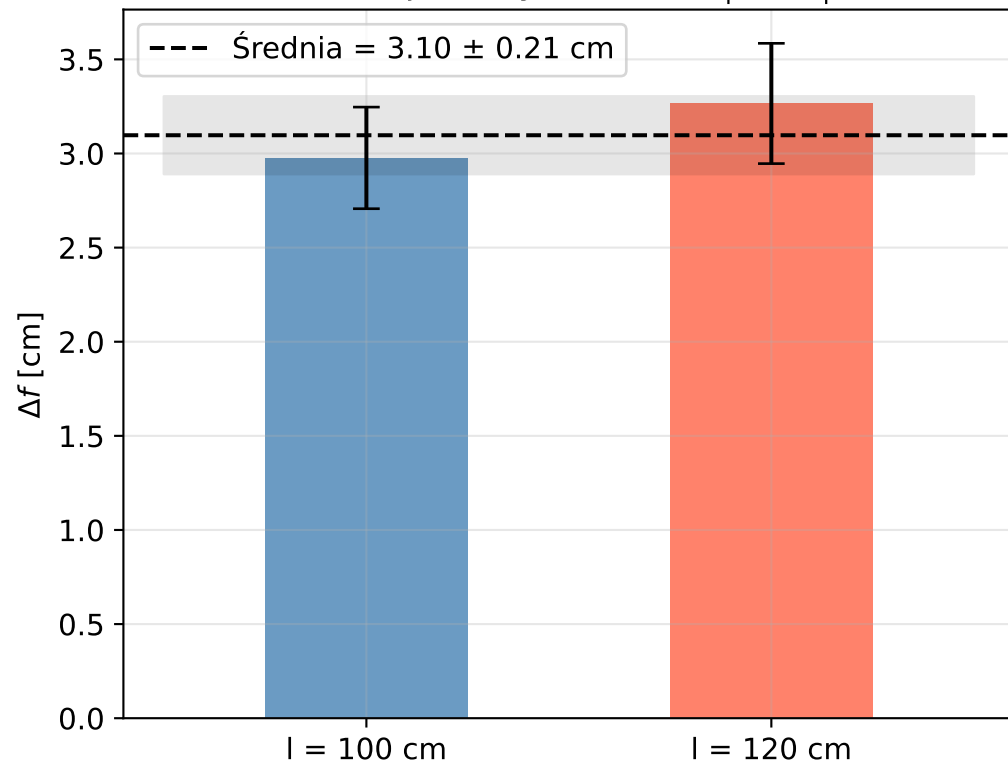
Aberracja sferyczna \Delta f = f_{\text{par}} - f_{\text{per}}
