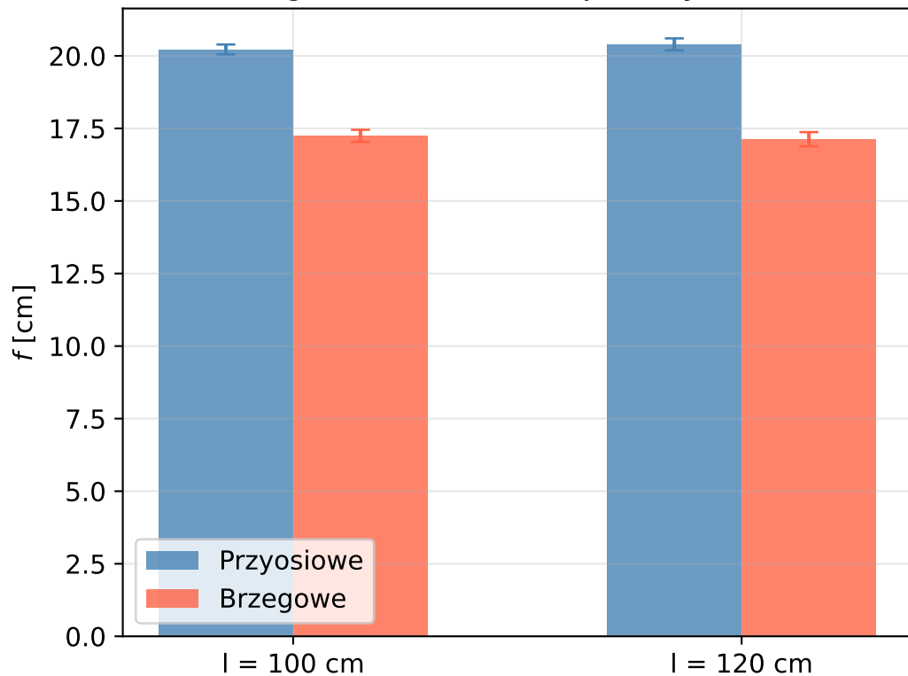
Ogniskowe – aberracja sferyczna
